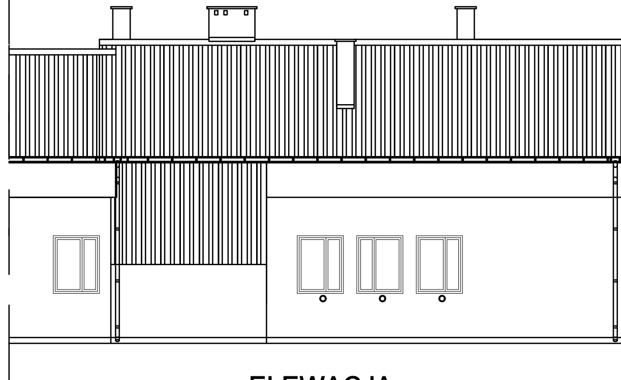
ELEWACJA POŁUDNIOWO-WSCHODNIA
